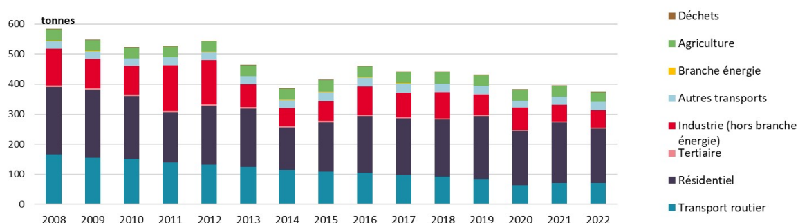
Figure 10. Evolution des émissions en particules PM10 (Source : Air Pays de la Loire)
