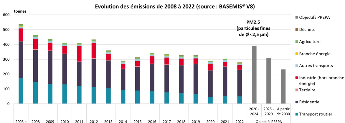
Figure 9. Evolution des émissions en particules fines PM2.5 et objectifs PREPA (Source : Air Pays de la Loire)
