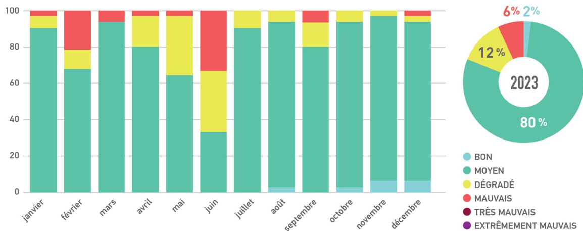
Figure 19. Distribution mensuelle des indices de qualité de l'air (Source : Air Pays de la Loire)
