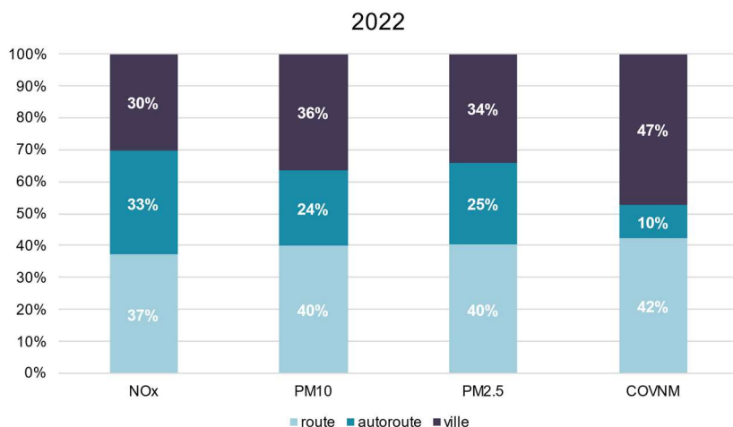
Figure 7. Répartition des émissions de polluants atmosphériques en 2022 dues au transport terrestre à l'échelle du Mans Métropole par type d'infrastructure (Source : Air Pays de la Loire)
