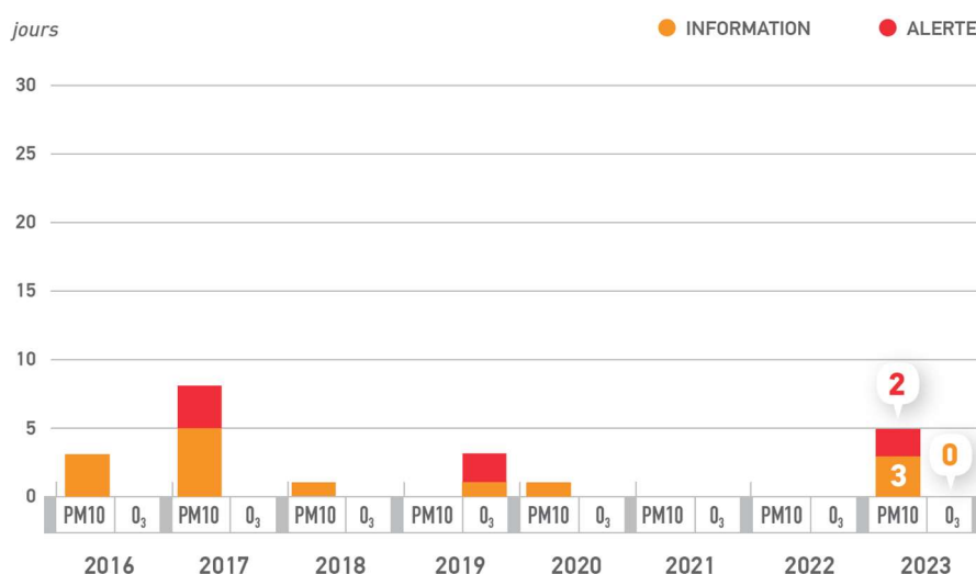
Figure 20. Historique du nombre de jours de procédure d'information ou d'alerte pour les particules PM10 et l'ozone sur le territoire du Mans Métropole (Source : Air Pays de la Loire)
