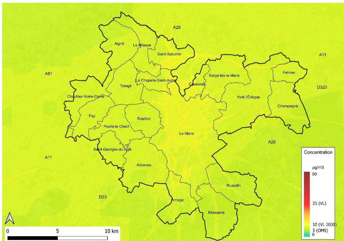
Figure 23. Concentration annuelle 2023 modélisée en particules PM2.5 (Source : Air Pays de la Loire)
